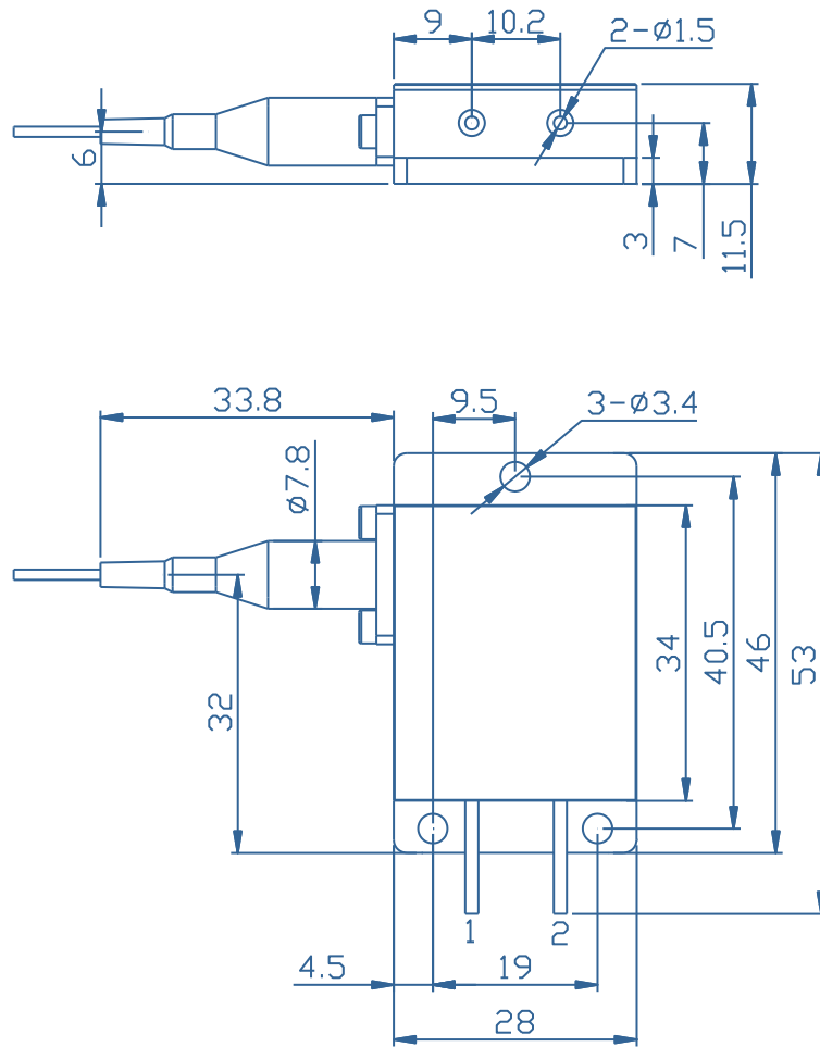
引脚功能分配 Pin-out Assignment
